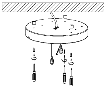
Takmontering
