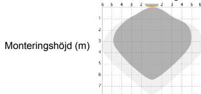
Takmontering
